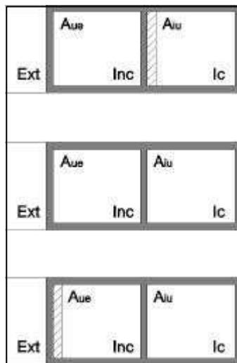
Figura E.6 Espacios habitables en contacto con espacios no habitables
