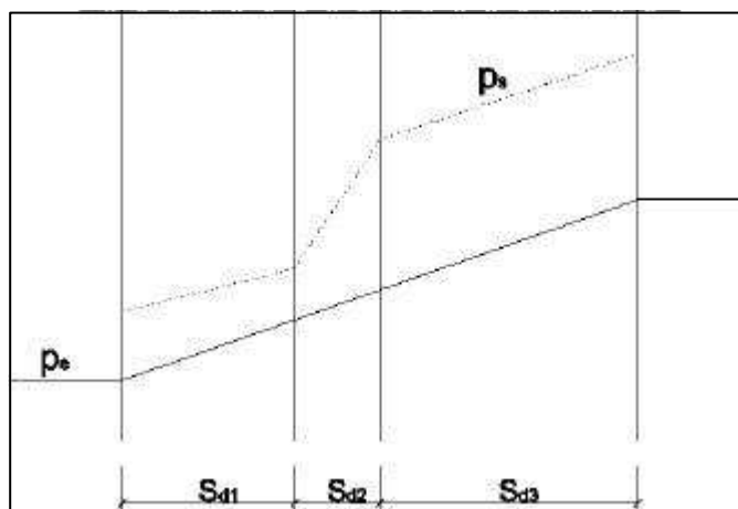
Figura H.1 Distribución de presiones de vapor de saturación y presiones de vapor en un elemento multicapa del edificio dibujada frente a la resistencia a presión de vapor de cada capa.
