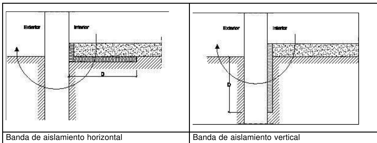
Figura E.1. Soleras con aislamiento perimetral
