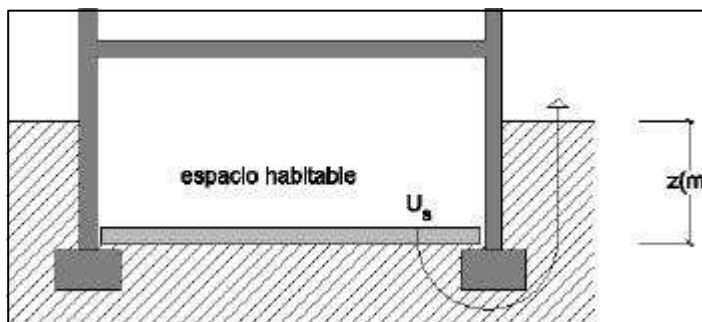
Figura E.2. Solera enterrada
